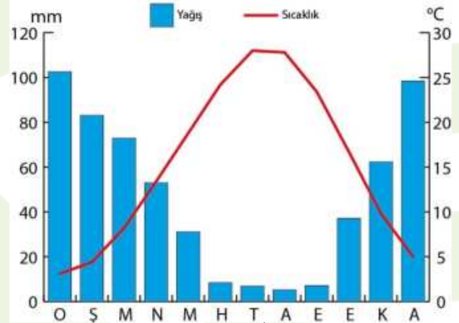
Gaziantep'in Sıcaklık ve Yağış Grafiđi
